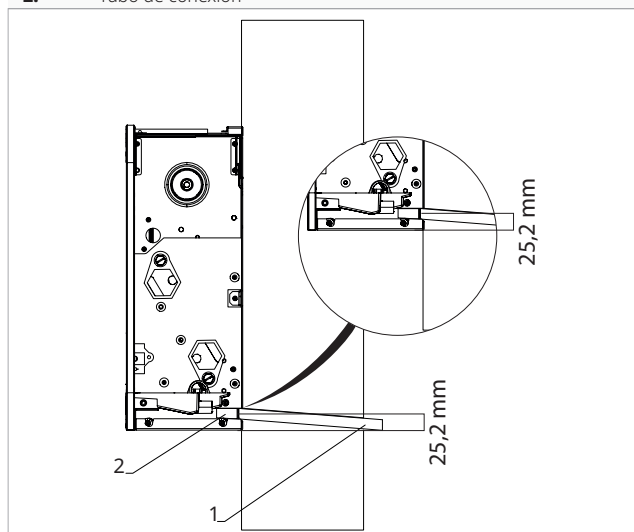
1. Tubería de drenaje 2. Tubo de conexión
