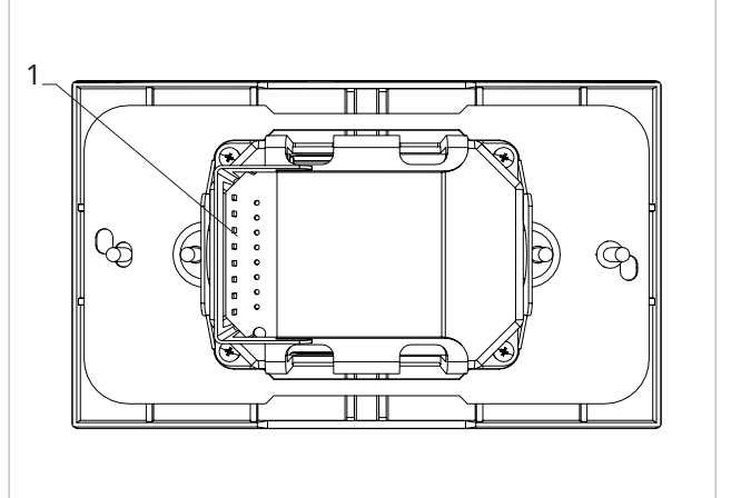
1. Bornier (Panneau vue postérieure)
