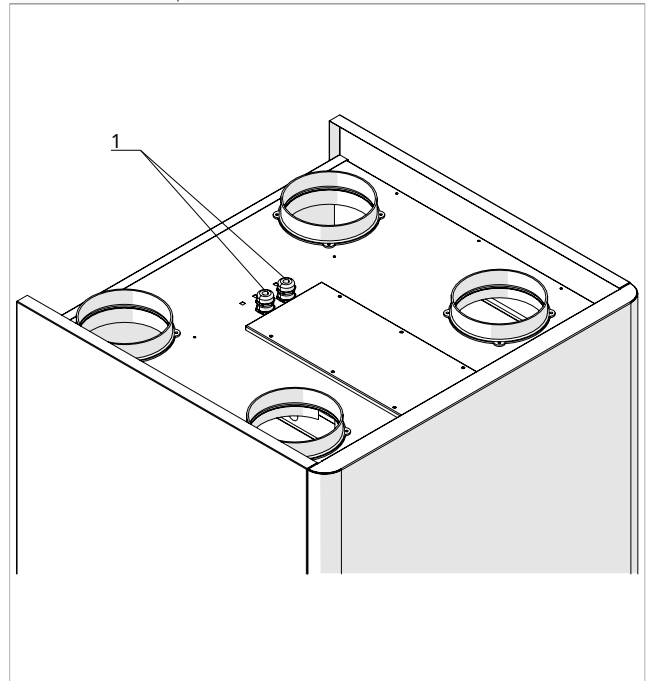
1. Presse-étoupe
