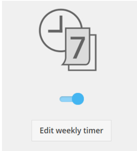
Afbeelding 19: week-timer aan/uit
