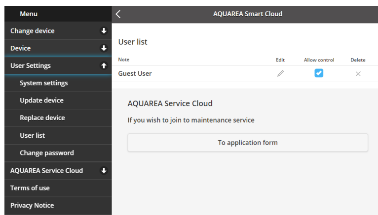
Afbeelding 32: Gebruikerslijst
