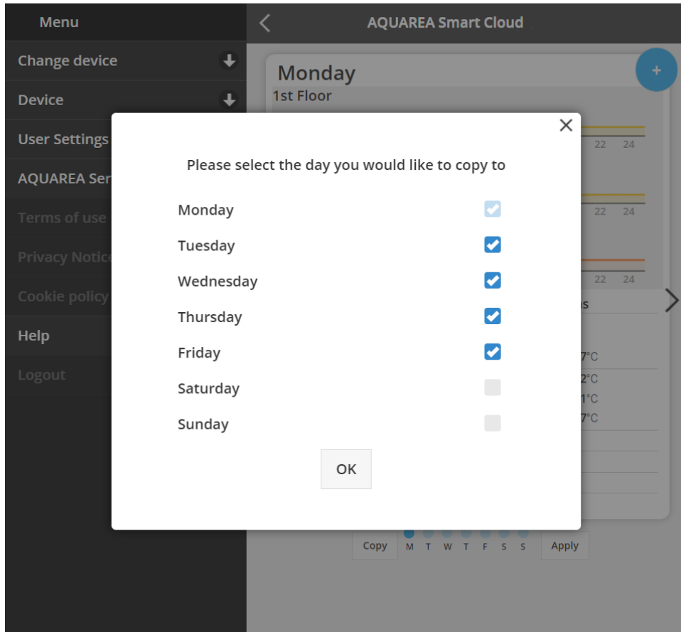
Afbeelding 21: menu 'Kopiëren'
