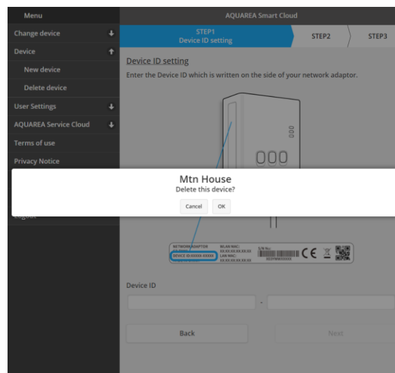
Afbeelding 28: Verwijder apparaat
