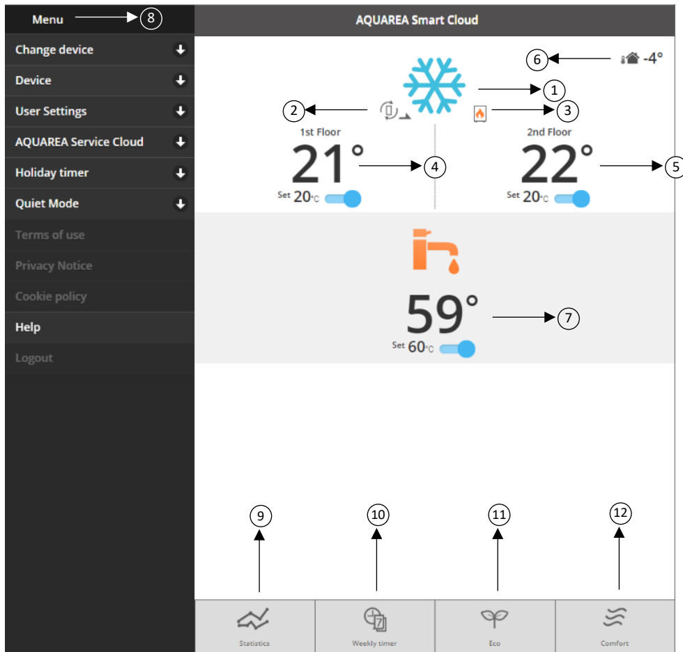
Afbeelding 14: bedieningscherm
