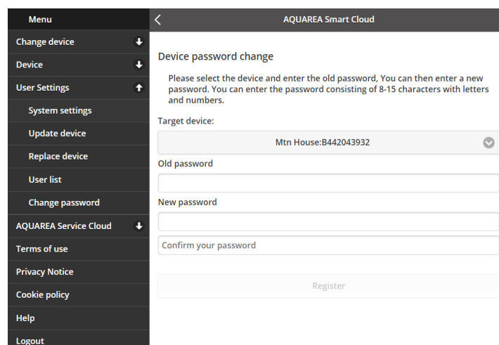
Afbeelding 34: Verander wachtwoord
