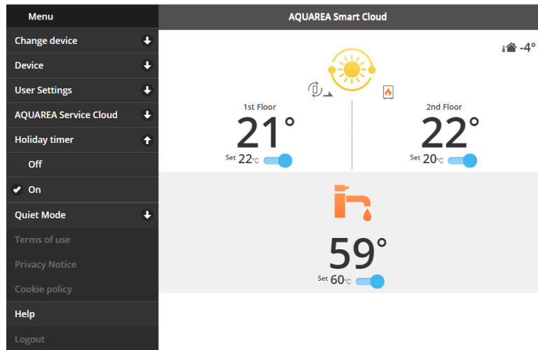
Afbeelding 37: Vakantie-timer
